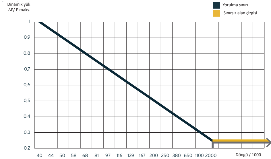
ŞEKİL 7.1 Yapı yorulması için en kötü durum senaryosu
