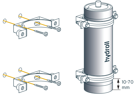
ŞEKİL 5.3 Önerilen kelepçe pozisyonları
