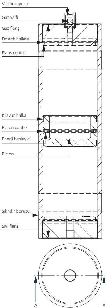
ŞEKİL 4.3 Bölüm A-A, M16x2 standart gaz valfi tipli akümülatör
