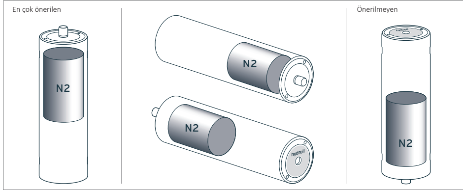
ŞEKİL 5.2 Montaj pozisyonları
