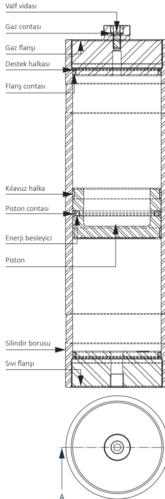
ŞEKİL 4.2 Bölüm A-A, M28x1,5 gaz valfi tipli akümülatör
