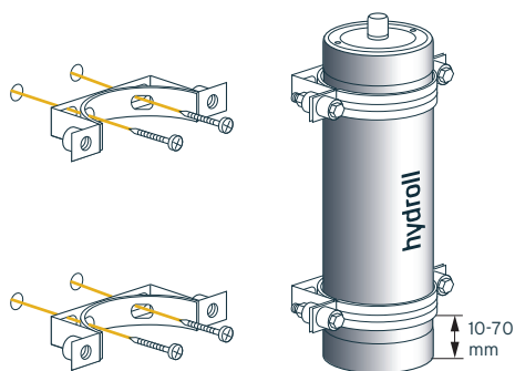
ФИГУРА 5.3 Препоръчани позиции на захващане
