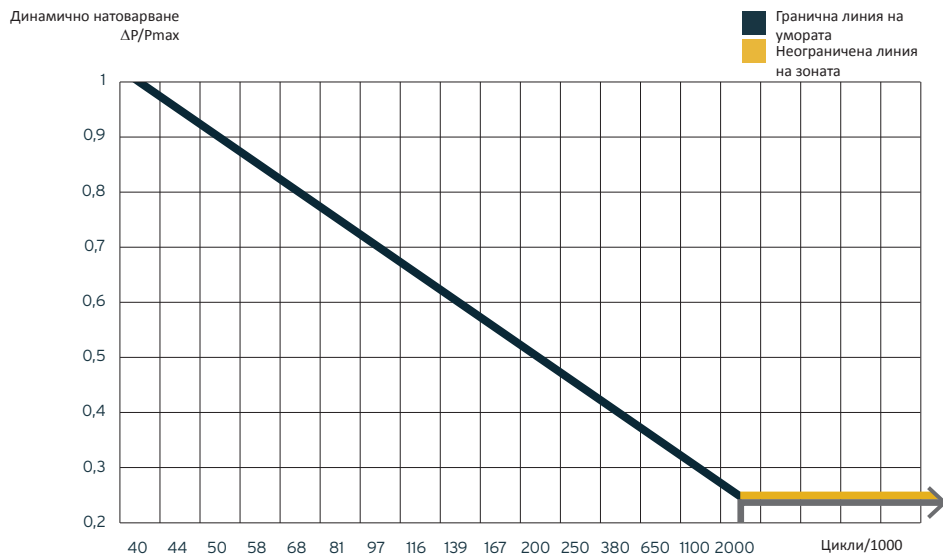
ФИГУРА 7.1 Умора на конструкцията в най-лошия случай
