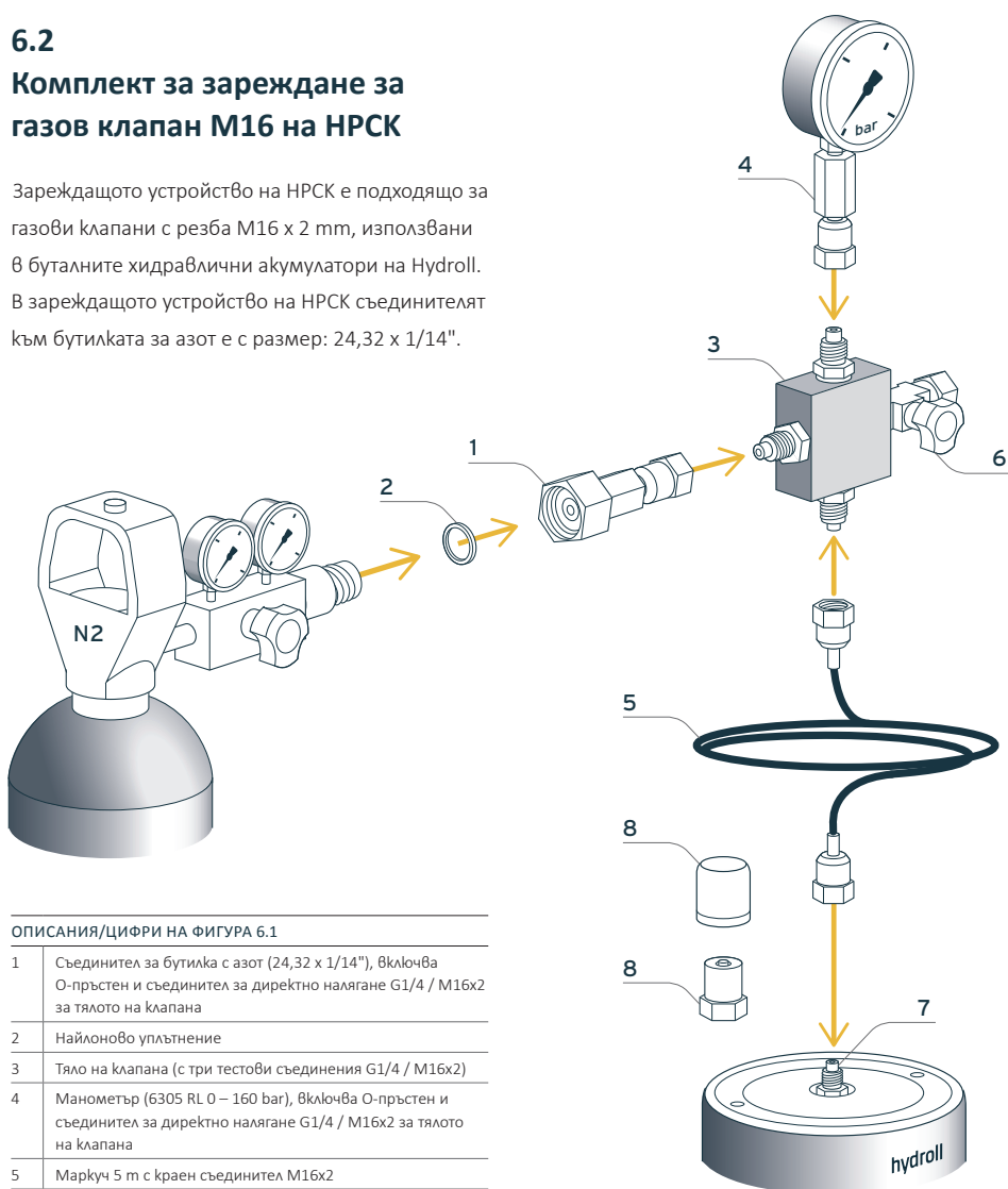
ФИГУРА 6.1 Комплект за зареждане за газов клапан M16 на НРСК, вижте описанията
