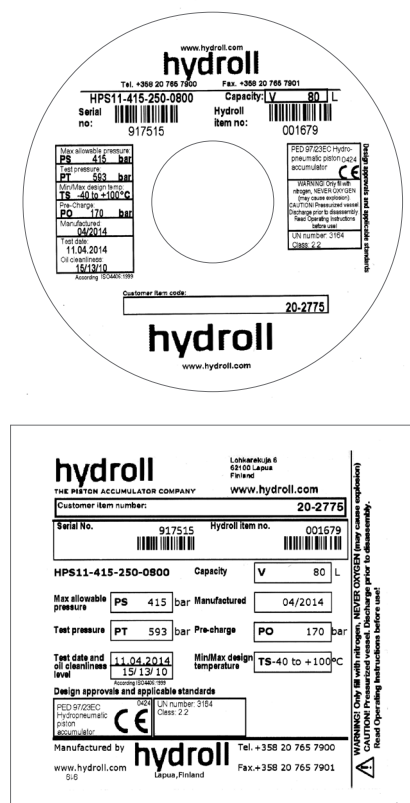
ФИГУРА 4.1 Примери на етикети на продукта
