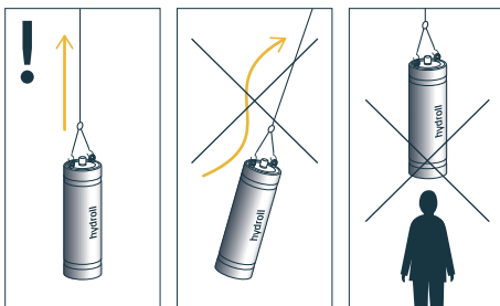
ФИГУРА 5.1 Точки на повдигане
